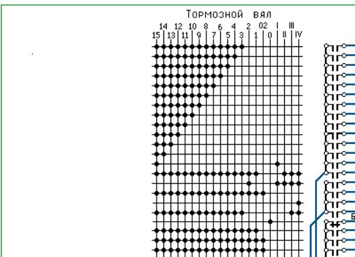
Контроллер машиниста 95-1 (96-2)
