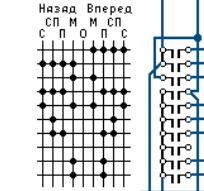
Реверсивно-селективный вал
